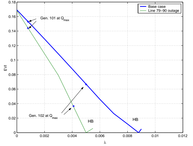
Fig. 16. Eigenvalue index for the IEEE 50-machine system, Case I.
